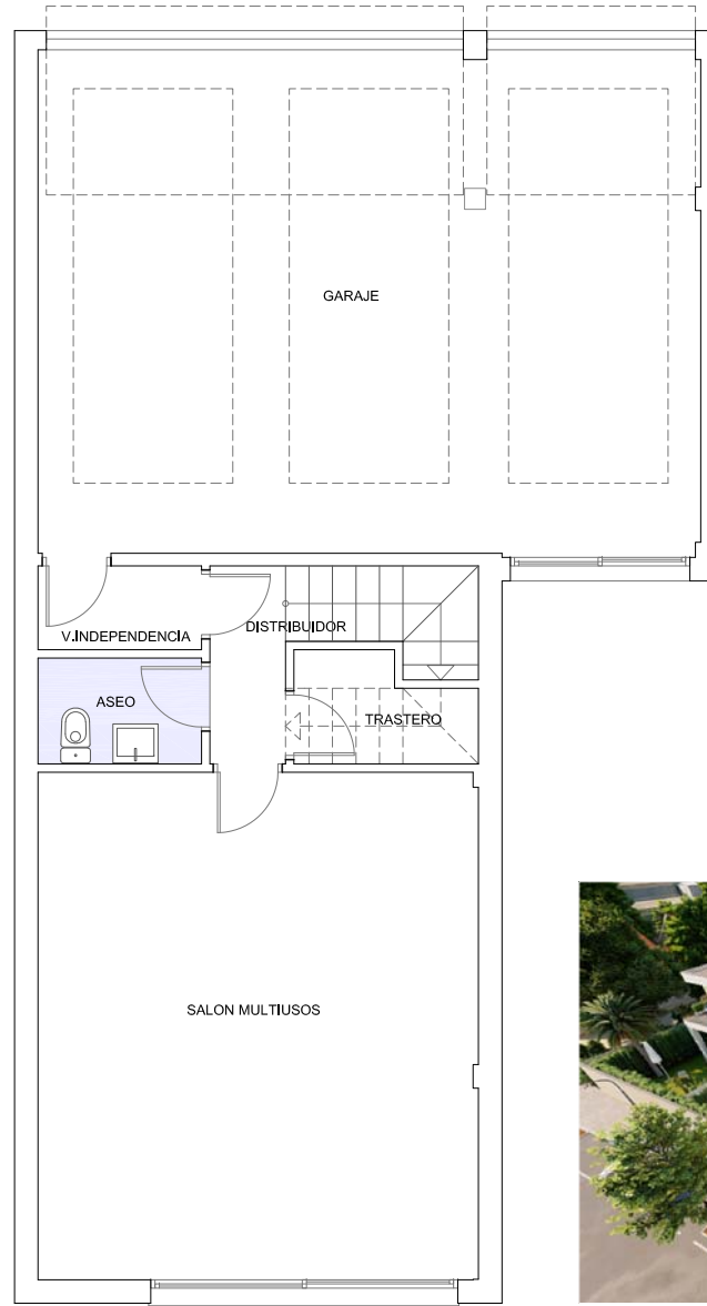
PLANTA SOTANO
