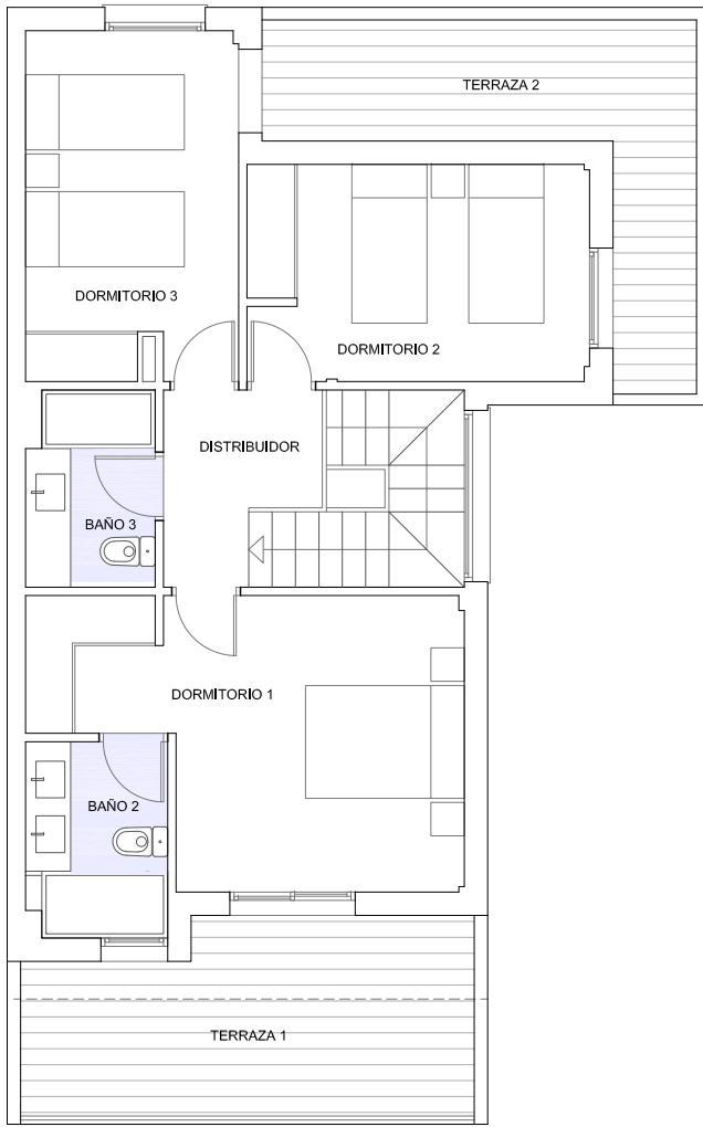
PLANTA PRIMERA
