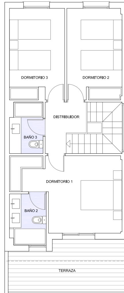
PLANTA PRIMERA
