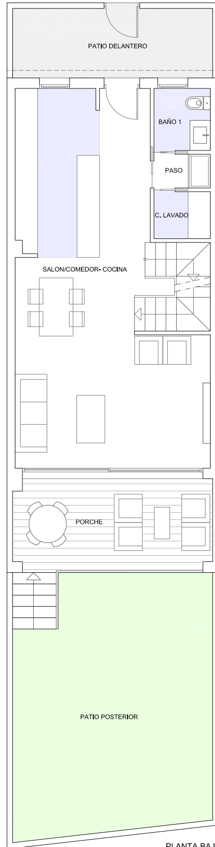
PLANTA BAJA
